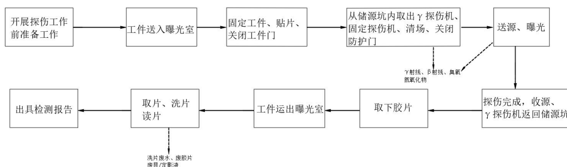
图 9-10 \gamma 射线探伤工艺流程及产污环节图
