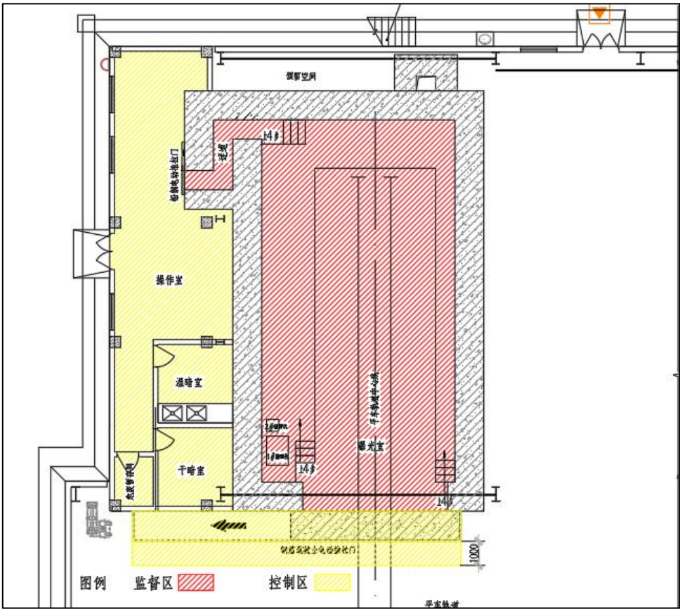
图 10-1 项目两区划分示意图
