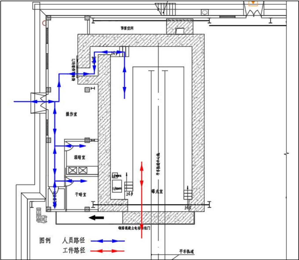
图 9-11 X 射线/γ 射线探伤工件及人员路径示意图
