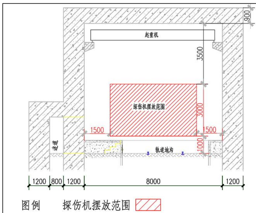
图 9-6 X/γ射线探伤机摆放范围立面图
