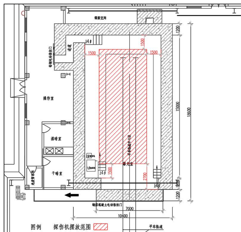
图 9-5 X/γ射线探伤机摆放范围俯视图
