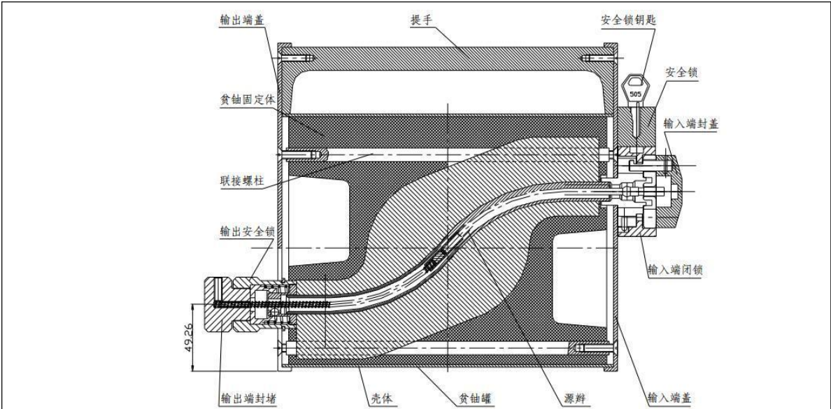
图 9-9 γ 射线探伤机内部结构图
