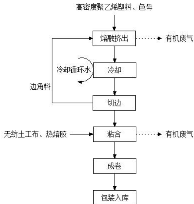
图 2-1 土工膜生产工艺流程及产污节点图
