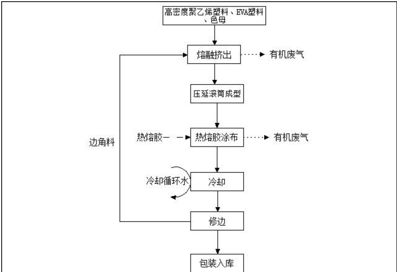
图 2-2 防水板生产工艺流程及产污节点图
